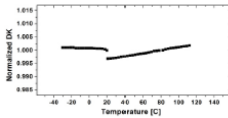
IPC-650 2.5.5.5.1 (加圧)
