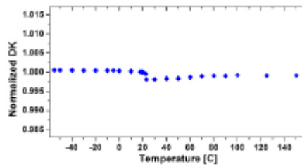
IPC-650 2.5.5.5 (加圧)
